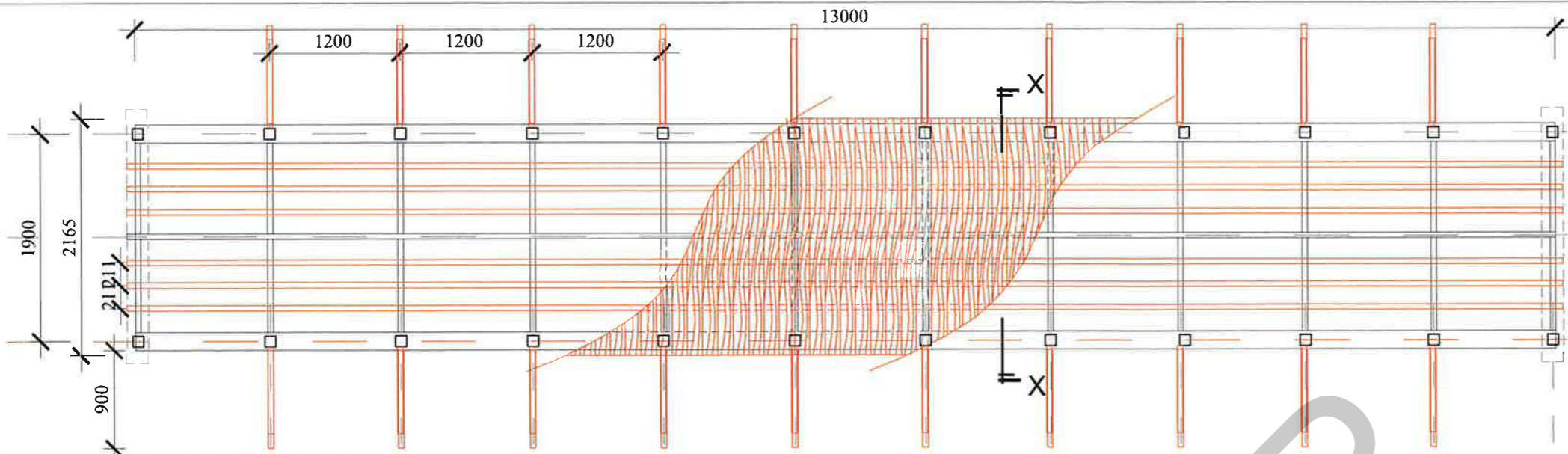
PLAN JAMBATAN L01/M48 Scale = 1 : 100
