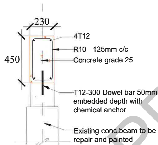
DETAIL E Scale : n.t.s
