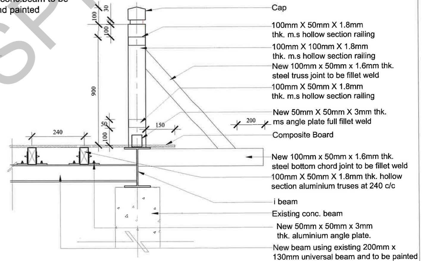
DETAIL E Scale : n.t.s
