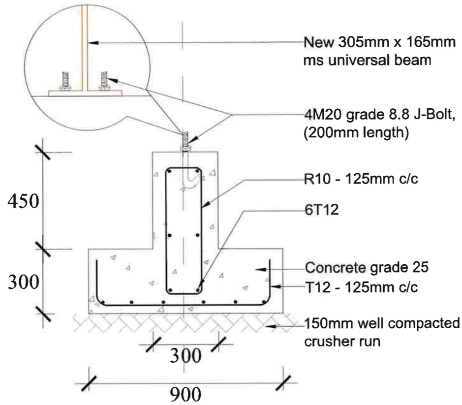
DETAIL J Scale : n.t.s
