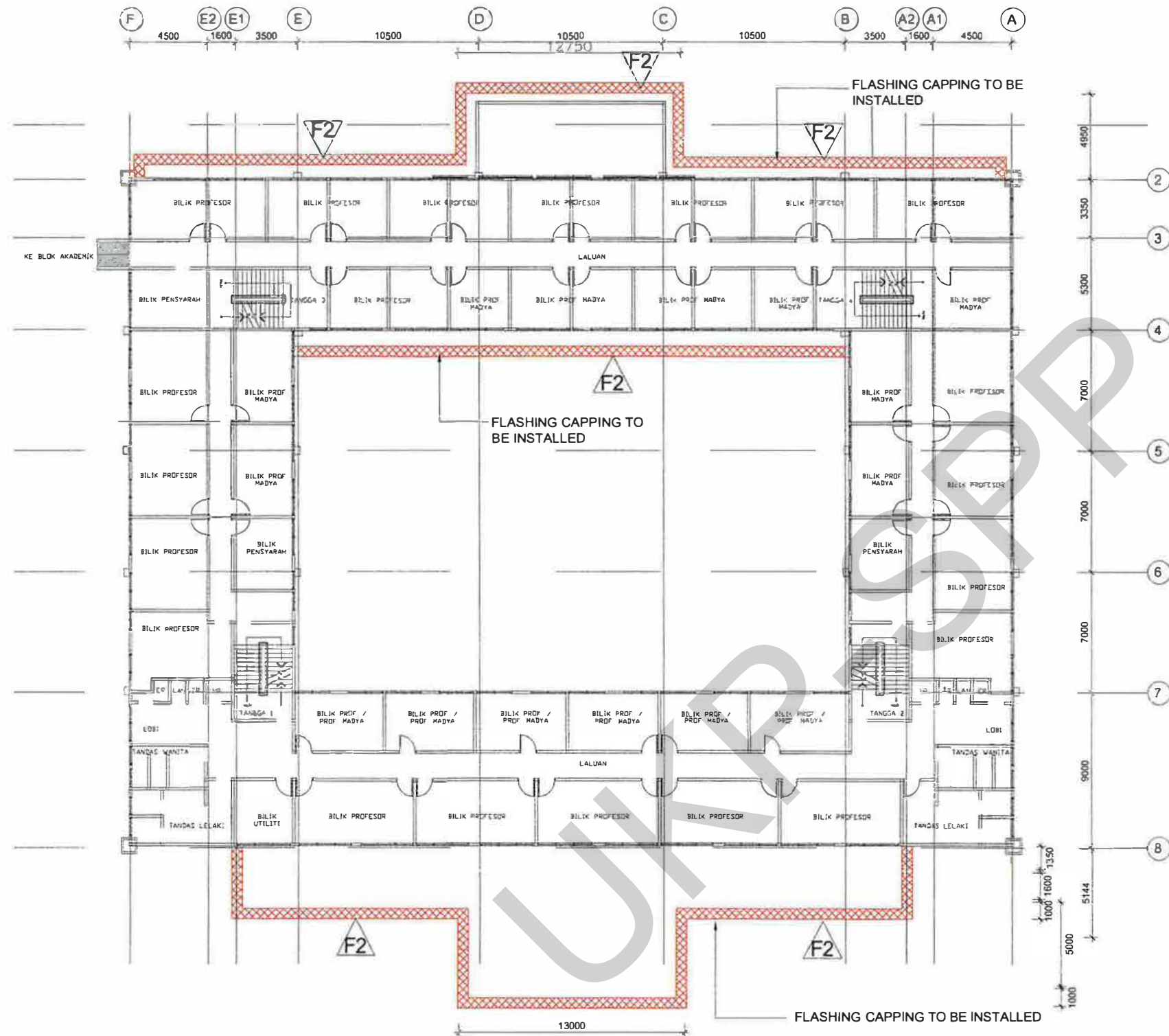
SEKOLAH KEJURUTERAAN AWAM BLOK M46 PELAN LANTAI ARAS 1 skala: 1 : 300
