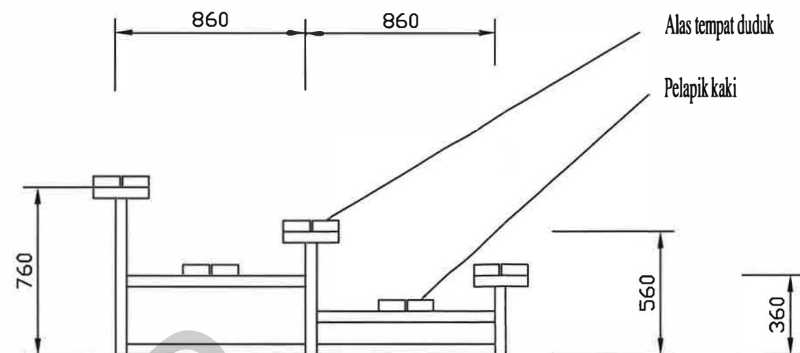
PDG. SISI
