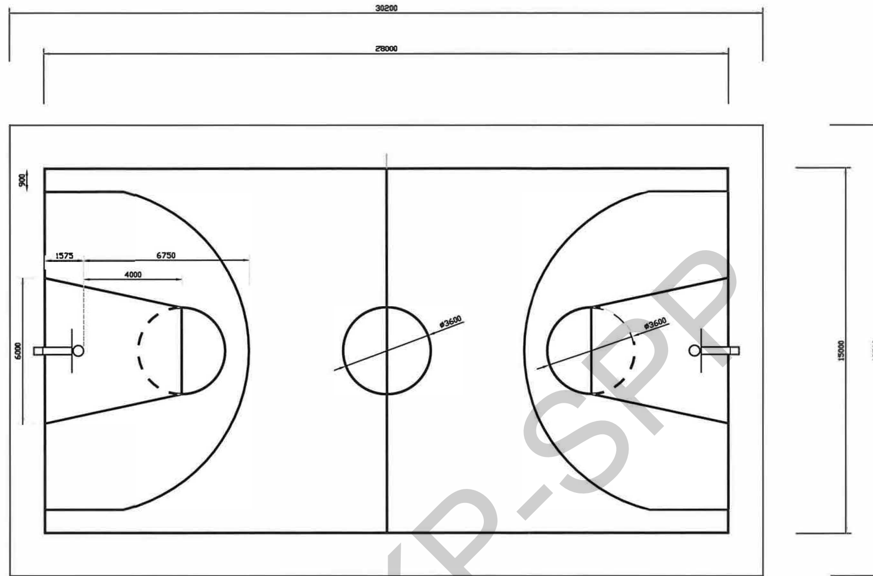
PELAN
